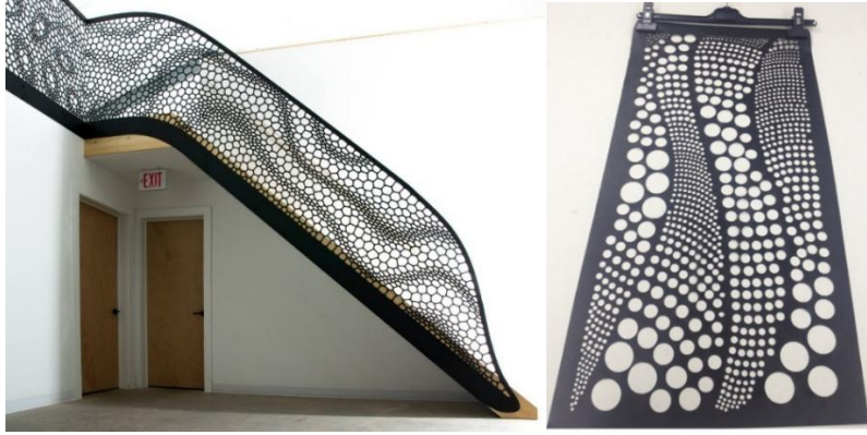
Görsel 16. Soldaki görsel iç mimaride tasarlanan Korollaria korkuluk, Parametrik tasarım yöntemi ile belli algoritmalarla oluşan, lazerle kesilmiş çelik korkuluk. Sağdaki görsel ise Parametrik tasarım anlayışı ile Korollaria korkuluktan esinlenerek yapılan lazer kesim yüzeyi
